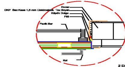
2 DETAYI
